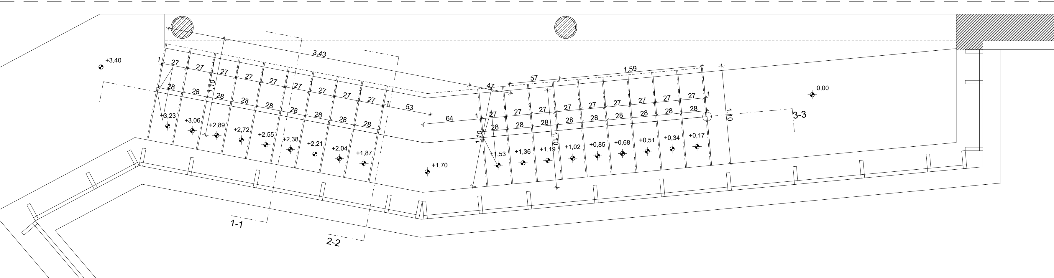
FÖLDSZINTI LÉPCSŐ ALAPRAJZ M1:25
