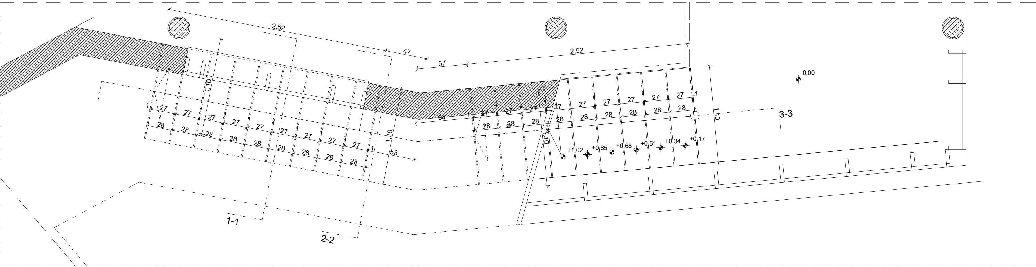
FÖLDSZINTI LÉPCSŐ ALAPRAJZ M1:25
