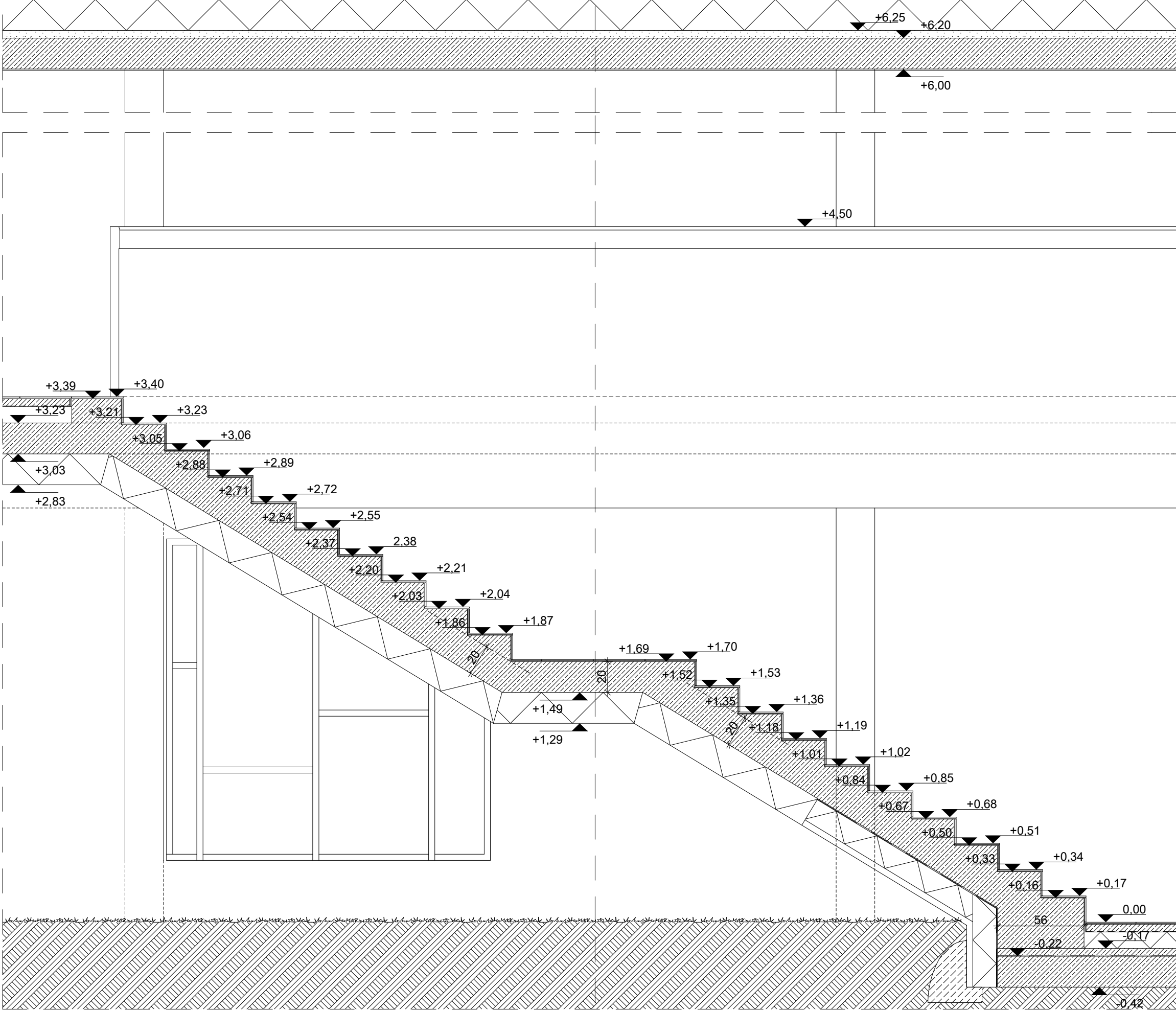
3-3 LÉPCSŐ METSZET M1:25
