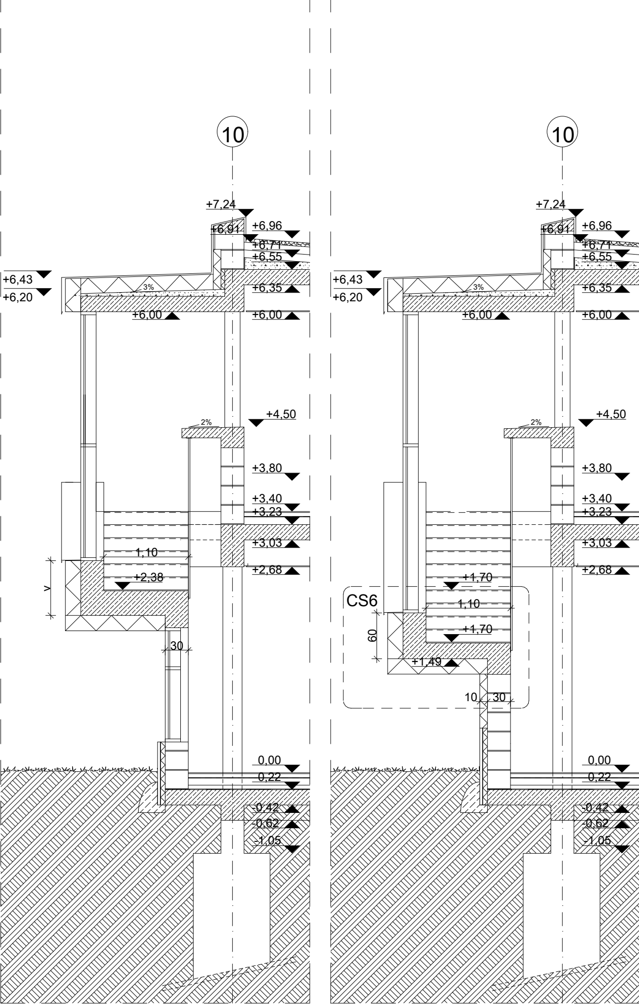
1-1 LÉPCSŐ METSZET M1:25
