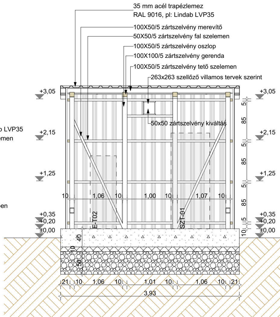
B-B metszet
